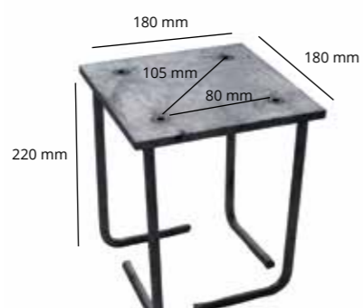
Ancrage au sol
