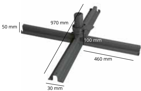
Pied de dalles
