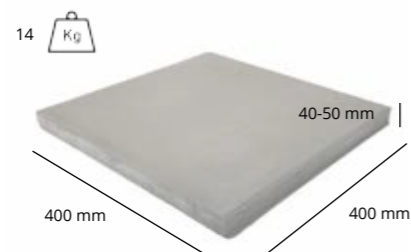
Le socle convient pour 4 dalles de 40 à 40 cm
